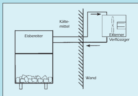
Luftgekühlte Ausführung mit externem Verflüssiger
